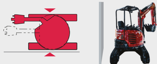
Escavação lateral de valas bem próxima à parede sem sair do alinhamento.
